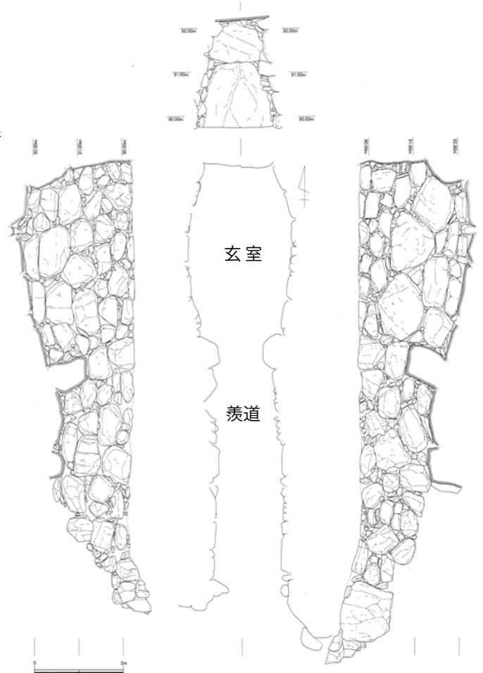
桂坪古墳 石室実測図 (S=1/120)
