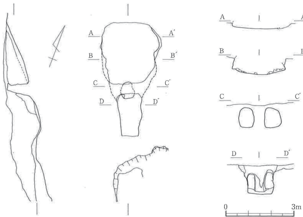
南山 9C 号窑 窑体实测图
