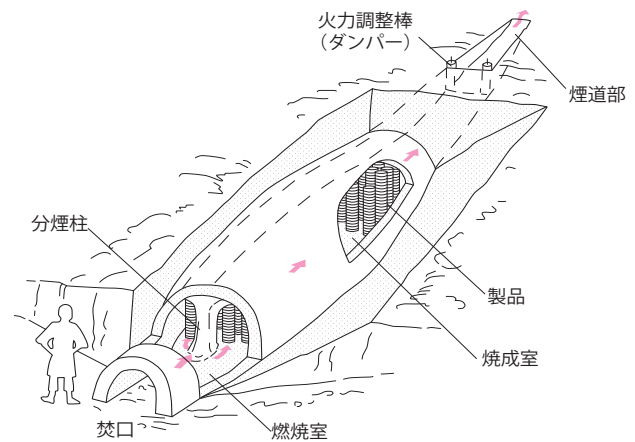
窖窯模式図
