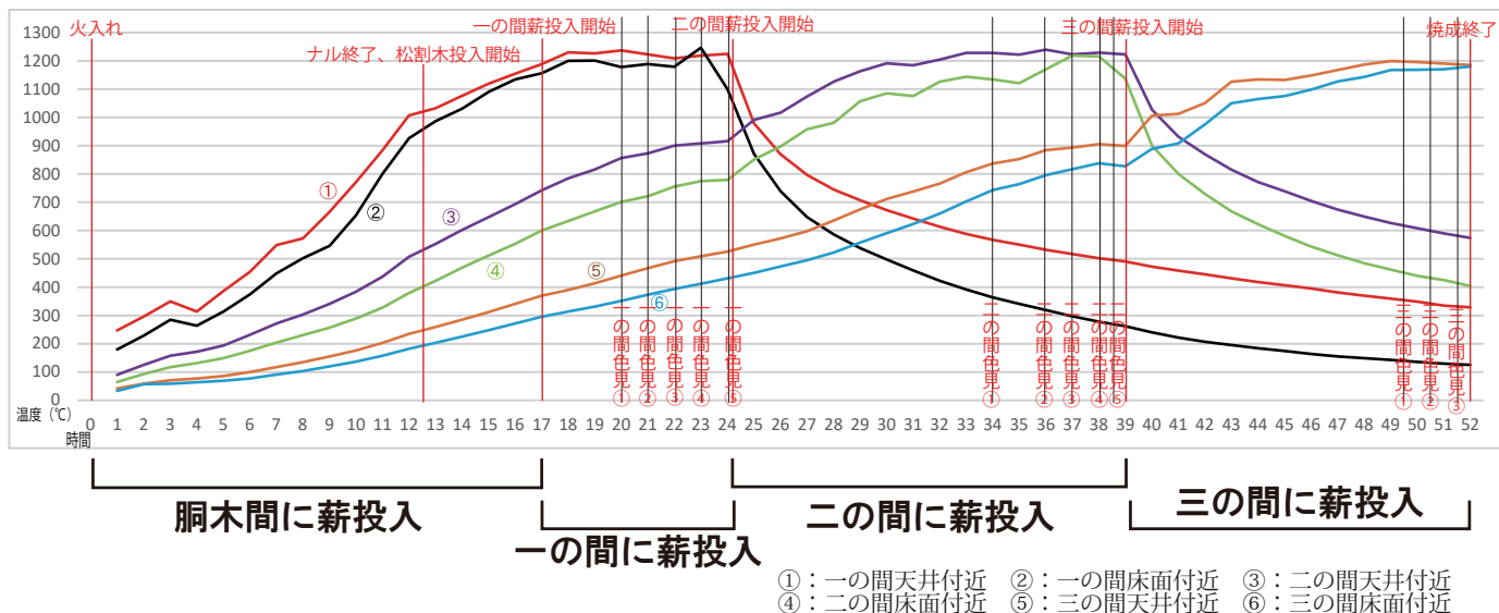
焼成室別の温度変化
