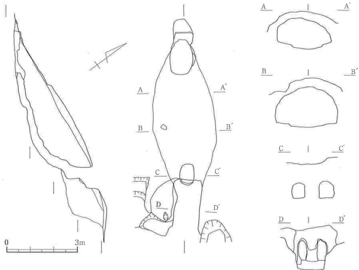
南山 9A 号窑 窑体实测图
