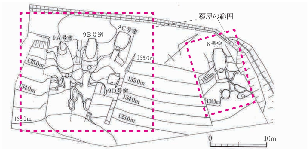
南山 8・9号窯跡 窯体配置図
