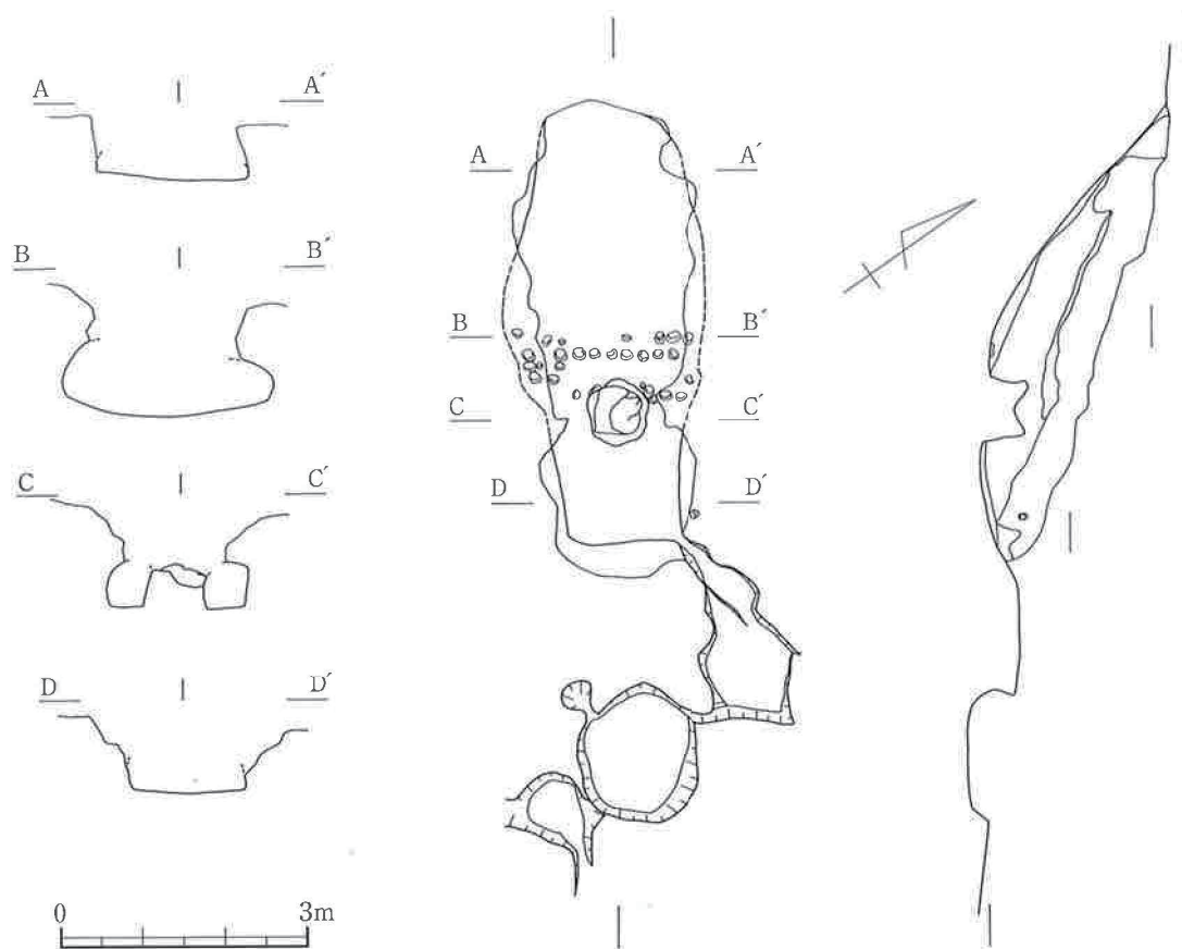
南山 8号窯 窯体実測図
