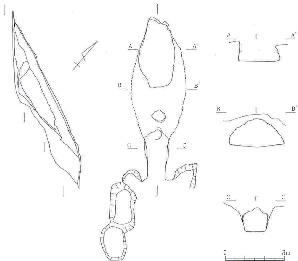
南山 9B 号窑 窑体实测图
